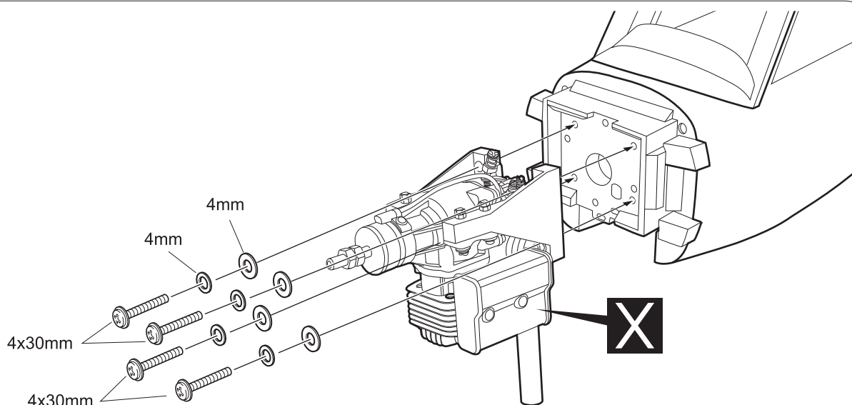
DLE 20
