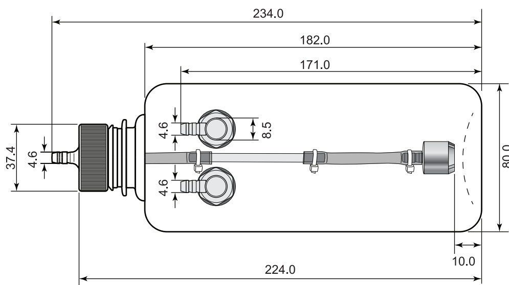
&lt; Top View &gt;
